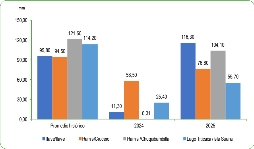
GRÁFICO N°71 PERÚ: PROMEDIO DE LAS PRECIPITACIONES EN LA VERTIENTE DEL LAGO TITICACA DICIEMBRE 2024 – 2025 Milímetros (mm)
