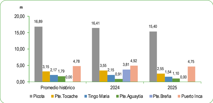
GRÁFICO N°62 PERÚ: CAUDAL PROMEDIO DE LOS RÍOS DE LA ZONA CENTRO DE LA VERTIENTE DEL ATLÁNTICO DICIEMBRE 2024 – 2025 Metro (m)
