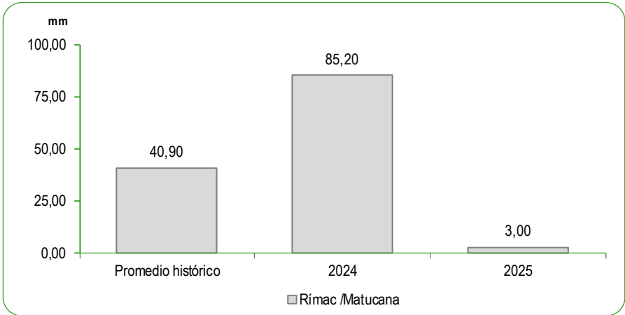
GRÁFICO N°66 PERÚ: PROMEDIO DE LAS PRECIPITACIONES EN LA ZONA CENTRO DE LA VERTIENTE DEL PACÍFICO DICIEMBRE 2024 – 2025 Milímetros (mm)
