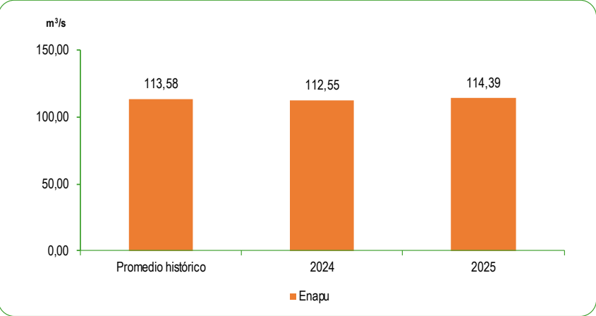
GRÁFICO N°61 PERÚ: CAUDAL PROMEDIO DE LOS RÍOS DE LA ZONA NORTE DE LA VERTIENTE DEL ATLÁNTICO DICIEMBRE 2024 – 2025 Metro cúbico por segundo (m³/s)
