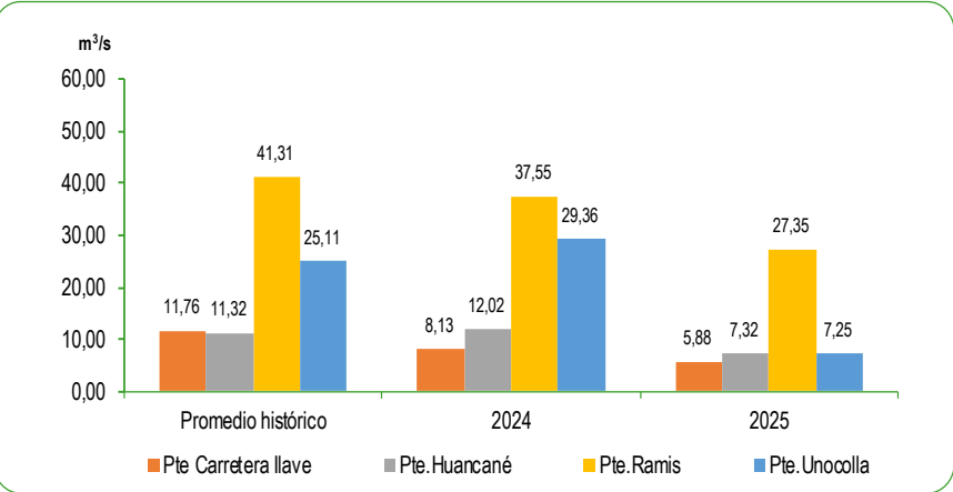
GRÁFICO N°64 PERÚ: CAUDAL PROMEDIO DE LOS RÍOS DE LA VERTIENTE DEL LAGO TITICACA DICIEMBRE 2024 – 2025 Metro cúbico por segundo (m³/s)
