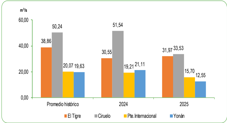
GRÁFICO N°58 PERÚ: CAUDAL PROMEDIO DE LOS RÍOS DE LA ZONA NORTE DE LA VERTIENTE DEL PACÍFICO DICIEMBRE 2024 - 2025 Metro cúbico por segundo (m³/s)
