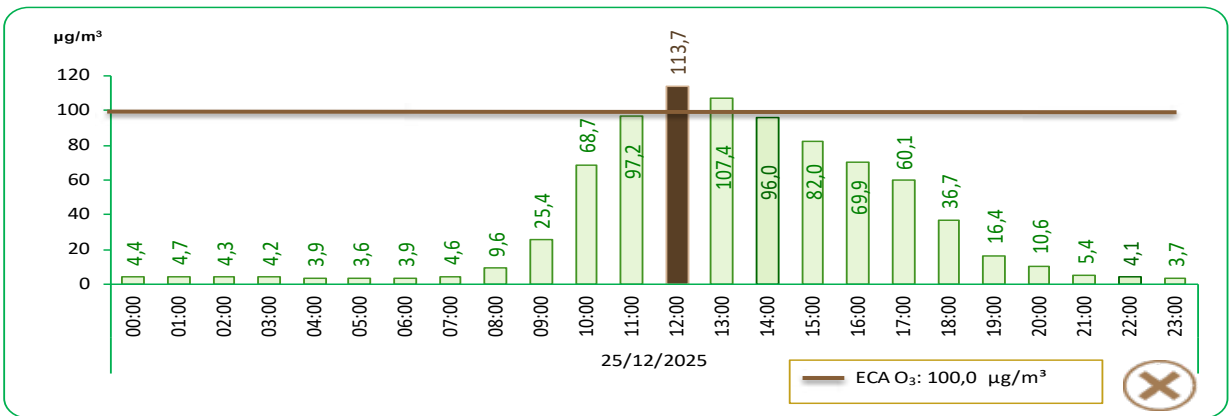
GRÁFICO N°38 LIMA METROPOLITANA: VALOR DIARIO DEL OZONO TROPOSFÉRICO (O 3 ), EN LA ESTACIÓN DE MEDICIÓN DE SAN JUAN DE LURIGANCHO – DICIEMBRE 2025
