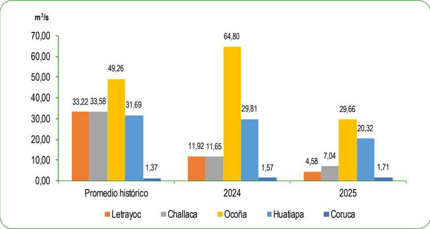
GRÁFICO N°60 PERÚ: CAUDAL PROMEDIO DE LOS RÍOS DE LA ZONA SUR DE LA VERTIENTE DEL PACÍFICO DICIEMBRE 2024 – 2025 Metro cúbico por segundo (m³/s)
