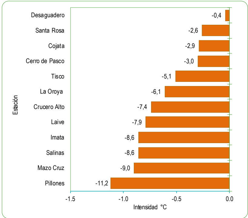
GRÁFICO N°74 PERÚ: MAYOR INTENSIDAD REGISTRADA DE LAS HELADAS METEOROLÓGICAS DICIEMBRE 2025 Temperatura bajo cero grados
