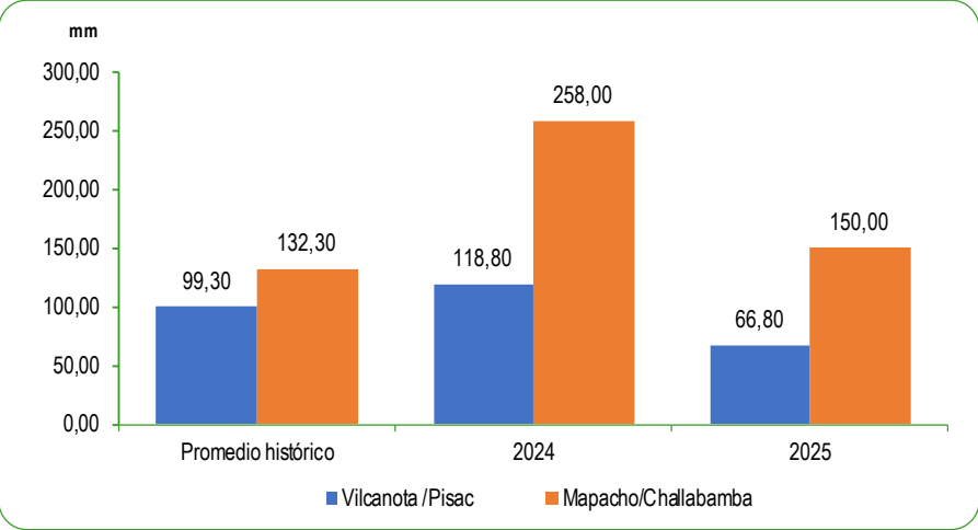
GRÁFICO N°70 PERÚ: PROMEDIO DE LAS PRECIPITACIONES EN LA ZONA SUR DE LA VERTIENTE DEL ATLÁNTICO DICIEMBRE 2023 - 2024 Milímetros (mm)
