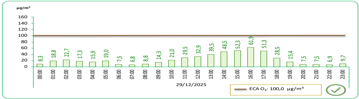
GRÁFICO N°34 LIMA METROPOLITANA: VALOR DIARIO DEL OZONO TROPOSFÉRICO (O 3 ), EN LA ESTACIÓN DE MEDICIÓN DE SAN BORJA – DICIEMBRE 2025
