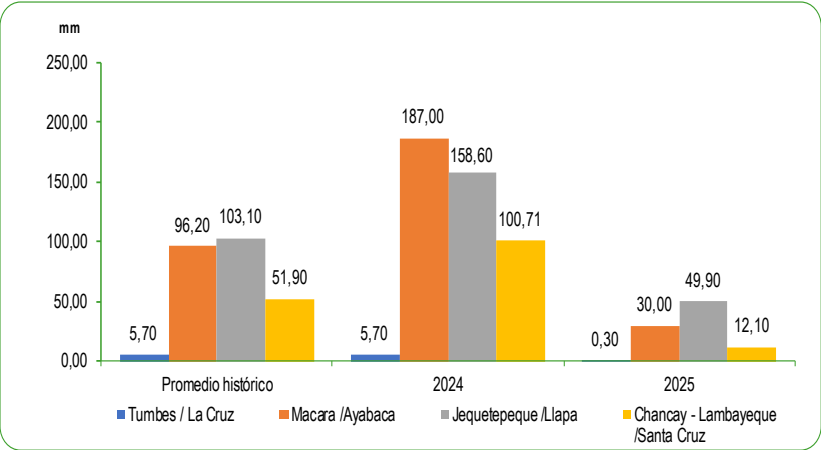
GRÁFICO N°65 PERÚ: PROMEDIO DE LAS PRECIPITACIONES EN LA ZONA NORTE DE LA VERTIENTE DEL PACÍFICO DICIEMBRE 2024 – 2025 Milímetros (mm)
