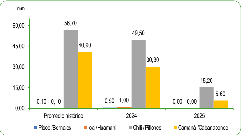
GRÁFICO N°67 PERÚ: PROMEDIO DE LAS PRECIPITACIONES EN LA ZONA SUR DE LA VERTIENTE DEL PACÍFICO DICIEMBRE 2024 - 2025 Milímetros (mm)
