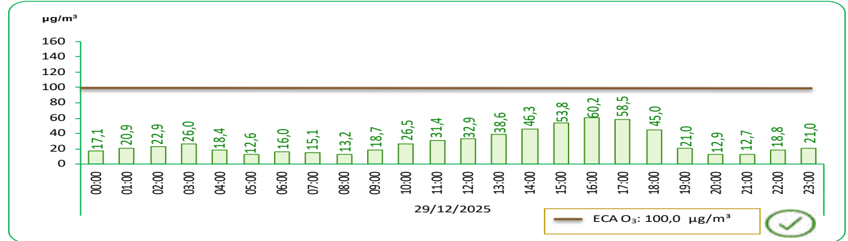
GRÁFICO N°35 LIMA METROPOLITANA: VALOR DIARIO DEL OZONO TROPOSFÉRICO (O 3 ), EN LA ESTACIÓN DE MEDICIÓN DE CAMPO DE MARTE – DICIEMBRE 2025
