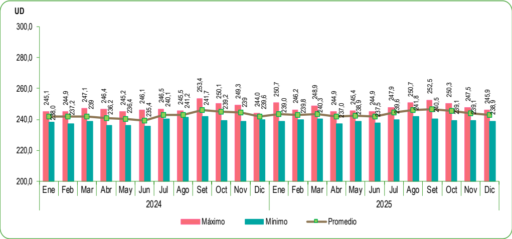
GRÁFICO N°41 PERÚ: VIGILANCIA DELOZONO ATMOSFÉRICO EN LA ESTACIÓN VAG MARCAPOMACOA DICIEMBRE 2025 – DICIEMBRE 2024 Unidades Dobson (UD)
