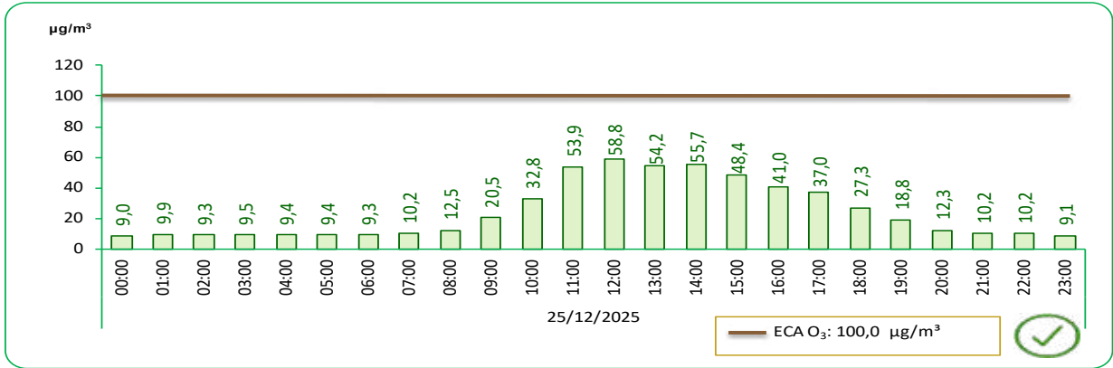
GRÁFICO N°37 LIMA METROPOLITANA: VALOR DIARIO DEL OZONO TROPOSFÉRICO (O 3 ), EN LA ESTACIÓN DE MEDICIÓN DE SANTA ANITA – DICIEMBRE 2025
