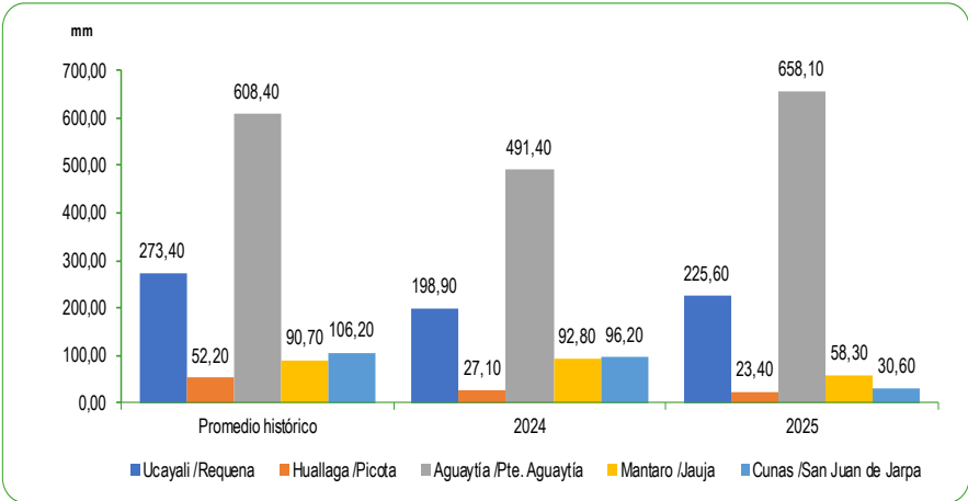
GRÁFICO N°69 PERÚ: PROMEDIO DE LAS PRECIPITACIONES EN LA ZONA CENTRO DE LA VERTIENTE DEL ATLÁNTICO DICIEMBRE 2024 – 2025 Milímetros (mm)
