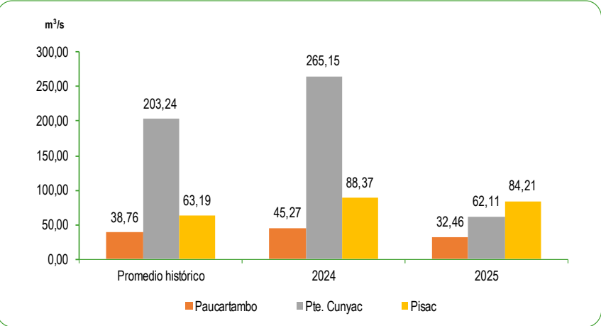
GRÁFICO N°63 PERÚ: CAUDAL PROMEDIO DE LOS RÍOS DE LA ZONA SUR DE LA VERTIENTE DEL ATLÁNTICO DICIEMBRE 2024 – 2025 Metro cúbico por segundo (m³/s)
