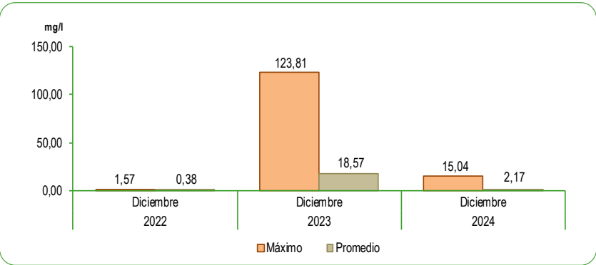
GRÁFICO N°48 LIMA METROPOLITANA: CONCENTRACIÓN DE ALUMINIO (Al) EN EL RÍO RÍMAC Mes: Diciembre 2022 - 2024 Miligramos por litro (mg/l)
