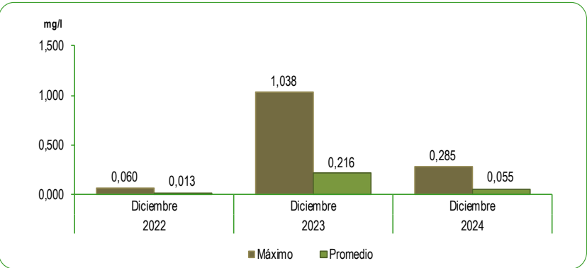
GRÁFICO N°44 LIMA METROPOLITANA: CONCENTRACIÓN DE PLOMO (Pb) EN EL RÍO RÍMAC Mes: Diciembre 2022 - 2024 Miligramos por litro (mg/l)
