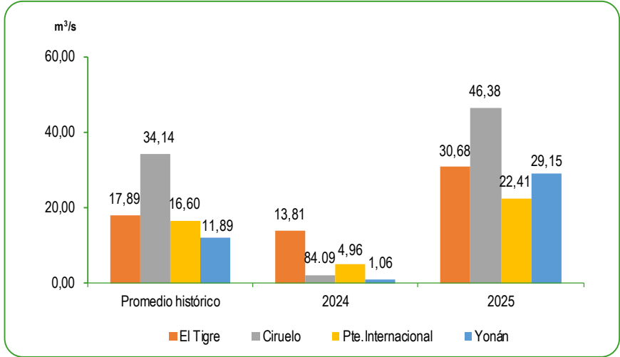
GRÁFICO N°58 PERÚ: CAUDAL PROMEDIO DE LOS RÍOS DE LA ZONA NORTE DE LA VERTIENTE DEL PACÍFICO NOVIEMBRE 2024 - 2025 Metro cúbico por segundo (m³/s)
