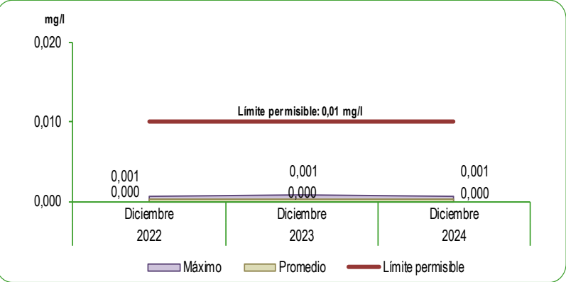
GRÁFICO N°45 LIMA METROPOLITANA: CONCENTRACIÓN DE PLOMO (Pb) EN LAS PLANTAS DE TRATAMIENTO 1 Y 2 DE SEDAPAL Mes: Diciembre 2022 - 2024 Miligramos por litro (mg/l)
