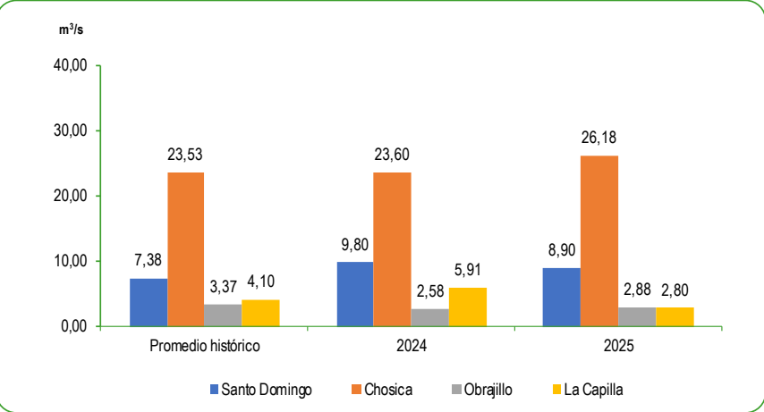
GRÁFICO N°59 PERÚ: CAUDAL PROMEDIO DE LOS RÍOS DE LA ZONA CENTRO DE LA VERTIENTE DEL PACÍFICO NOVIEMBRE 2024 – 2025 Metro cúbico por segundo (m³/s)
