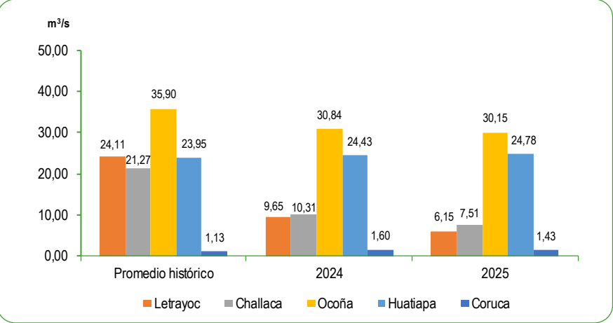
GRÁFICO N°60 PERÚ: CAUDAL PROMEDIO DE LOS RÍOS DE LA ZONA SUR DE LA VERTIENTE DEL PACÍFICO NOVIEMBRE 2024 – 2025 Metro cúbico por segundo (m³/s)
