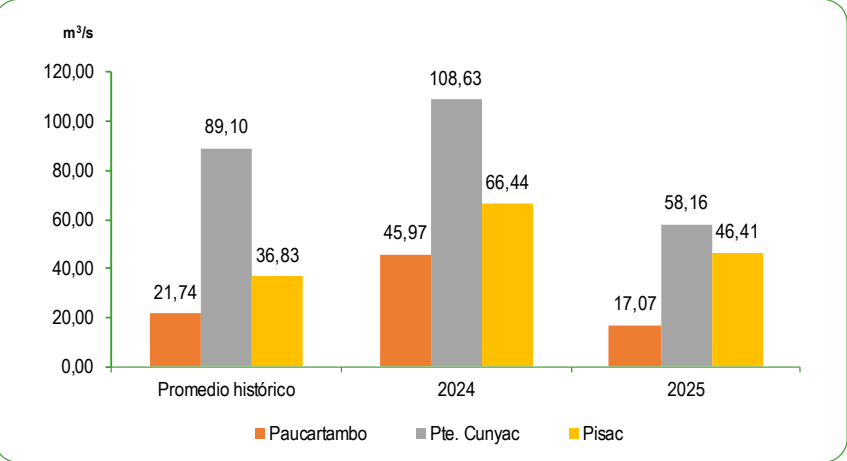
GRÁFICO N°63 PERÚ: CAUDAL PROMEDIO DE LOS RÍOS DE LA ZONA SUR DE LA VERTIENTE DEL ATLÁNTICO NOVIEMBRE 2024 – 2025 Metro cúbico por segundo (m³/s)
