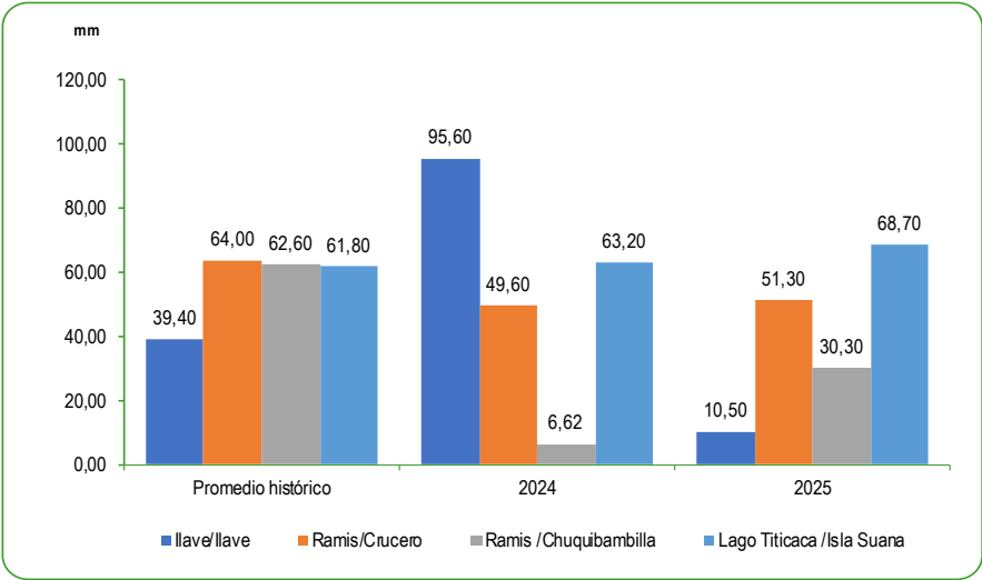
GRÁFICO N°71 PERÚ: PROMEDIO DE LAS PRECIPITACIONES EN LA VERTIENTE DEL LAGO TITICACA NOVIEMBRE 2024 – 2025 Milímetros (mm)
