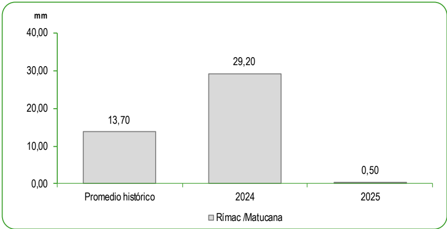
GRÁFICO N°66 PERÚ: PROMEDIO DE LAS PRECIPITACIONES EN LA ZONA CENTRO DE LA VERTIENTE DEL PACÍFICO NOVIEMBRE 2024 – 2025 Milímetros (mm)
