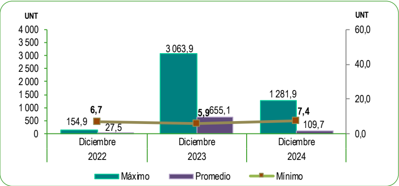
GRÁFICO N°54 LIMA METROPOLITANA: NIVELES DE TURBIEDAD EN EL RÍO RÍMAC Mes: Diciembre 2022 - 2024 Unidades Nefelométricas de Turbiedad (UNT)
