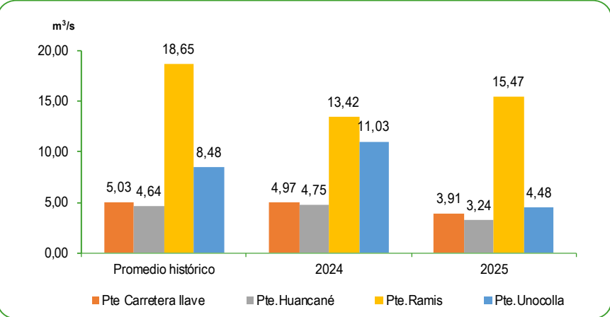
GRÁFICO N°64 PERÚ: CAUDAL PROMEDIO DE LOS RÍOS DE LA VERTIENTE DEL LAGO TITICACA NOVIEMBRE 2024 – 2025 Metro cúbico por segundo (m³/s)
