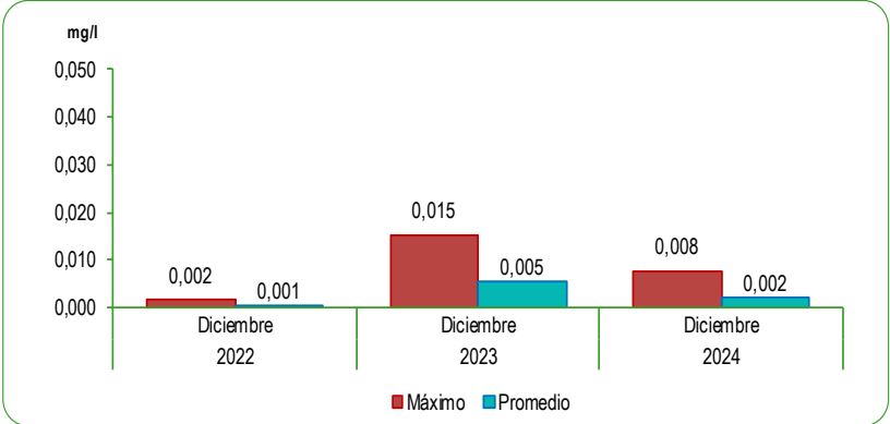
GRÁFICO N°46 LIMA METROPOLITANA: CONCENTRACIÓN DE CADMIO (Cd) EN EL RÍO RÍMAC Mes: Diciembre 2022 - 2024 Miligramos por litro (mg/l)
