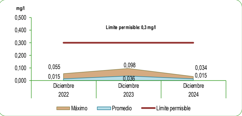
GRÁFICO N°43 LIMA METROPOLITANA: CONCENTRACIÓN DE HIERRO (Fe) EN LAS PLANTAS DE TRATAMIENTO 1 Y 2 DE SEDAPAL Mes: Diciembre 2022 - 2024 Miligramos por litro (mg/l)
