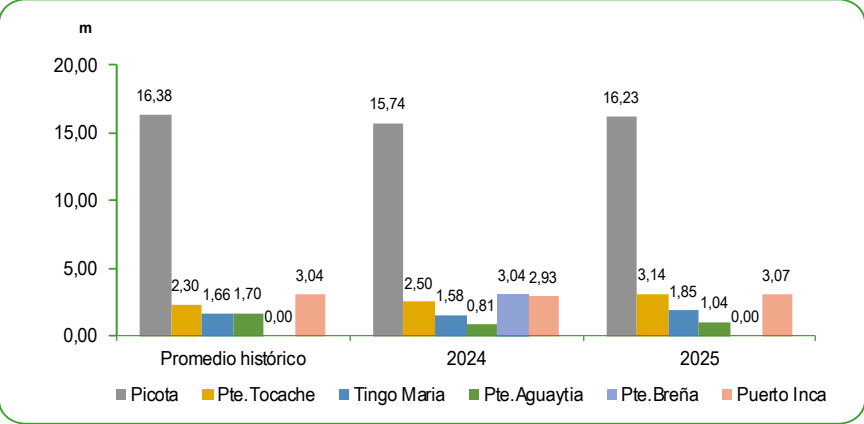
GRÁFICO N°62 PERÚ: CAUDAL PROMEDIO DE LOS RÍOS DE LA ZONA CENTRO DE LA VERTIENTE DEL ATLÁNTICO NOVIEMBRE 2024 – 2025 Metro (m)
