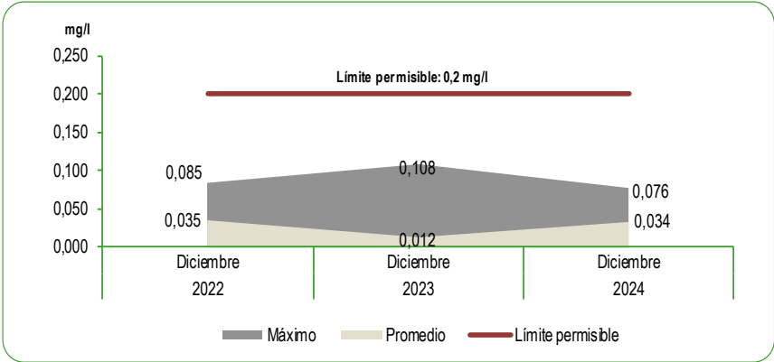
GRÁFICO N° 49 LIMA METROPOLITANA: CONCENTRACIÓN DE ALUMINIO (Al) EN LAS PLANTAS DE TRATAMIENTO 1 Y 2 DE SEDAPAL Mes: Diciembre 2022 - 2024 Miligramos por litro (mg/l)
