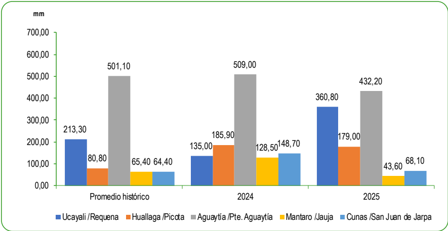
GRÁFICO N°69 PERÚ: PROMEDIO DE LAS PRECIPITACIONES EN LA ZONA CENTRO DE LA VERTIENTE DEL ATLÁNTICO NOVIEMBRE 2024 – 2025 Milímetros (mm)
