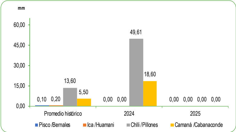
GRÁFICO N°67 PERÚ: PROMEDIO DE LAS PRECIPITACIONES EN LA ZONA SUR DE LA VERTIENTE DEL PACÍFICO NOVIEMBRE 2024 - 2025 Milímetros (mm)
