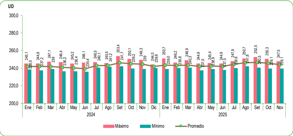
GRÁFICO N°41 PERÚ: VIGILANCIA DEL OZONO ATMOSFÉRICO EN LA ESTACIÓN VAG MARCAPOMACOA NOVIEMBRE 2025 – NOVIEMBRE 2024 Unidades Dobson (UD)
