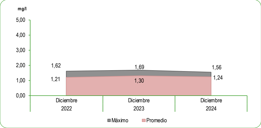
GRÁFICO N°51 LIMA METROPOLITANA: CONCENTRACIÓN DE MATERIA ORGÁNICA EXPRESADA COMO TOC EN LAS PLANTAS DE TRATAMIENTO 1 Y 2 DE SEDAPAL Mes: Diciembre 2022 - 2024 Miligramos por litro (mg/l)
