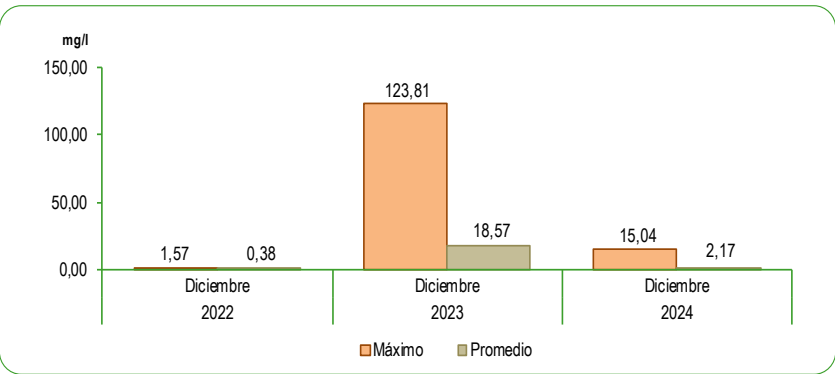
GRÁFICO N°51 LIMA METROPOLITANA: CONCENTRACIÓN DE ALUMINIO (Al) EN EL RÍO RÍMAC Mes: Diciembre 2022 - 2024 Miligramos por litro (mg/l)
