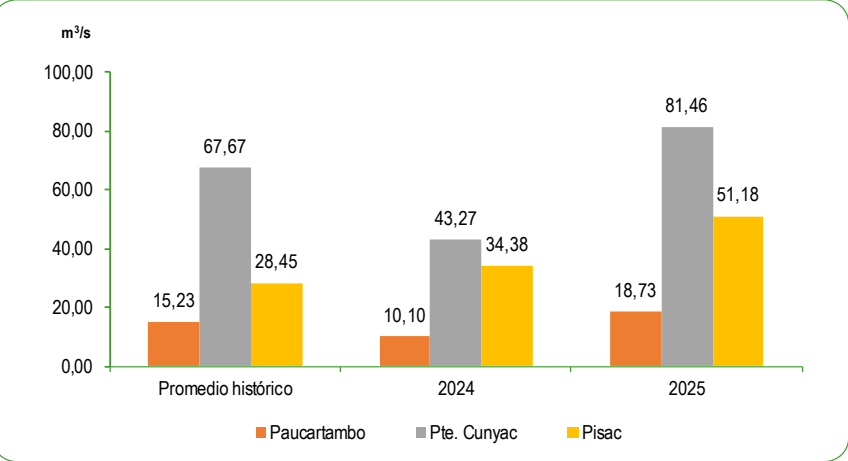
GRÁFICO N°66 PERÚ: CAUDAL PROMEDIO DE LOS RÍOS DE LA ZONA SUR DE LA VERTIENTE DEL ATLÁNTICO OCTUBRE 2024 – 2025 Metro cúbico por segundo (m³/s)
