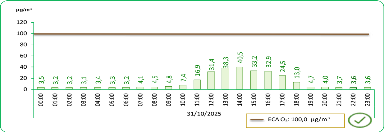
GRÁFICO N°40 LIMA METROPOLITANA: VALOR DIARIO DEL OZONO TROPOSFÉRICO (O 3 ), EN LA ESTACIÓN DE MEDICIÓN DE SAN JUAN DE LURIGANCHO – OCTUBRE 2025
