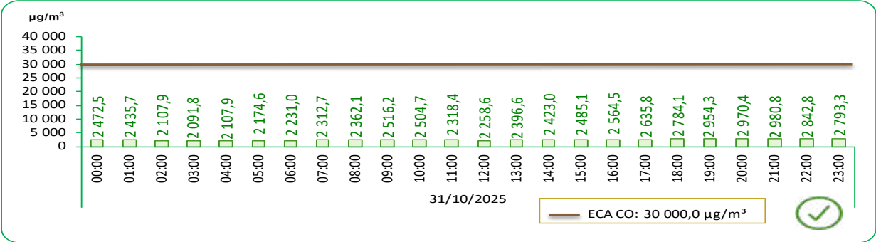
GRÁFICO N°29 LIMA METROPOLITANA: VALOR DIARIO DEL MONÓXIDO DE CARBONO (CO), EN LA ESTACIÓN DE MEDICIÓN DE PUENTE PIEDRA – OCTUBRE 2025
