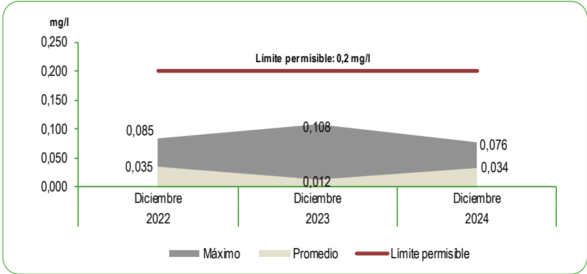
GRÁFICO N°52 LIMA METROPOLITANA: CONCENTRACIÓN DE ALUMINIO (Al) EN LAS PLANTAS DE TRATAMIENTO 1 Y 2 DE SEDAPAL Mes: Diciembre 2022 - 2024 Miligramos por litro (mg/l)
