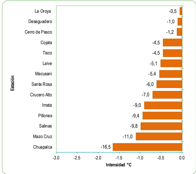
GRÁFICO N°77 PERÚ: MAYOR INTENSIDAD REGISTRADA DE LAS HELADAS METEOROLÓGICAS OCTUBRE 2025 Temperatura bajo cero grados
