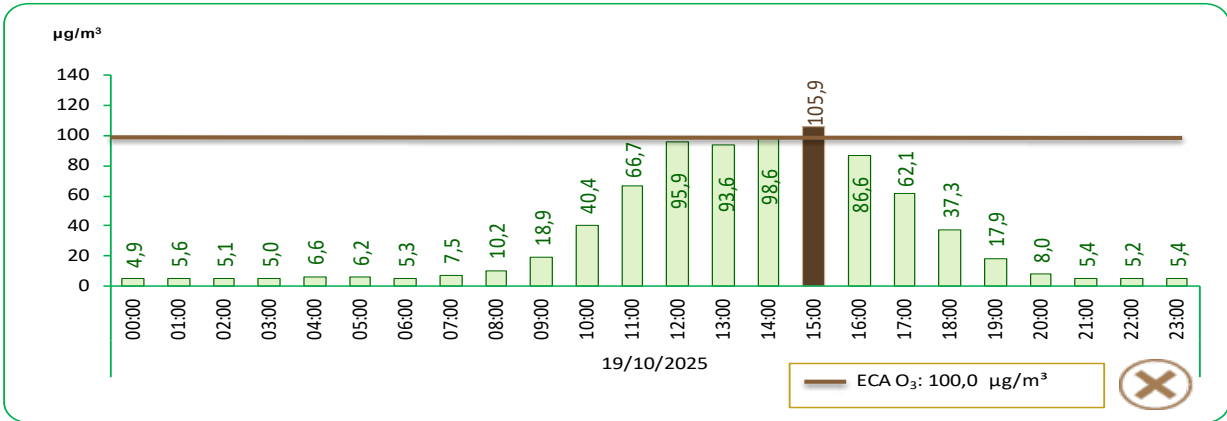
GRÁFICO N°41 LIMA METROPOLITANA: VALOR DIARIO DEL OZONO TROPOSFÉRICO (O 3 ), EN LA ESTACIÓN DE MEDICIÓN DE CERES – OCTUBRE 2025
