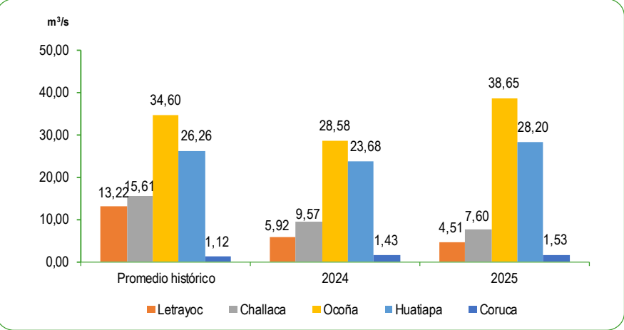
GRÁFICO N°63 PERÚ: CAUDAL PROMEDIO DE LOS RÍOS DE LA ZONA SUR DE LA VERTIENTE DEL PACÍFICO OCTUBRE 2024 – 2025 Metro cúbico por segundo (m³/s)
