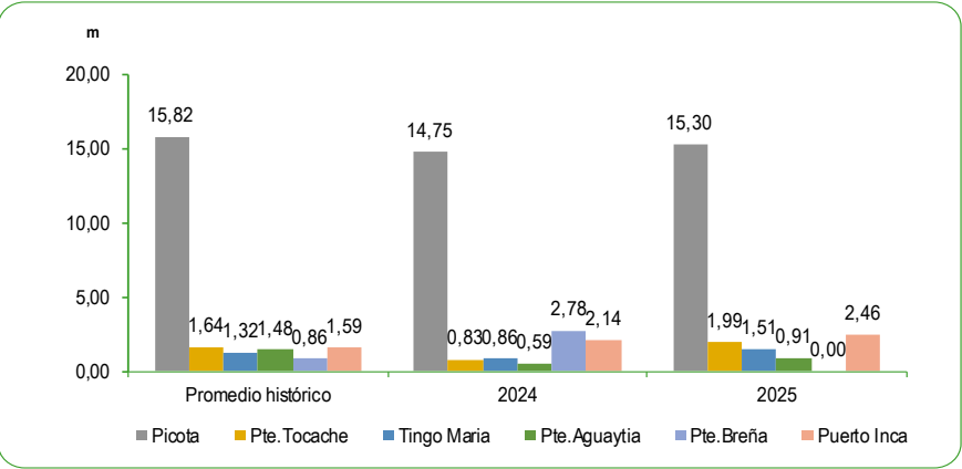
GRÁFICO N°65 PERÚ: CAUDAL PROMEDIO DE LOS RÍOS DE LA ZONA CENTRO DE LA VERTIENTE DEL ATLÁNTICO OCTUBRE 2024 – 2025 Metro (m)
