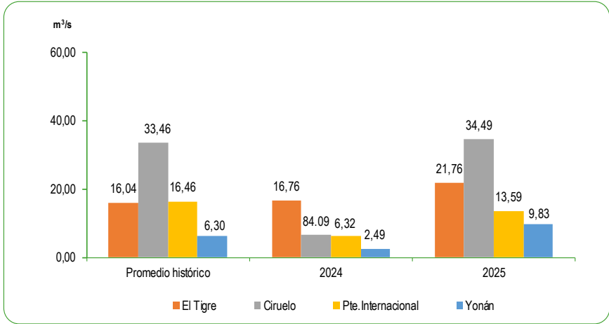
GRÁFICO N°61 PERÚ: CAUDAL PROMEDIO DE LOS RÍOS DE LA ZONA NORTE DE LA VERTIENTE DEL PACÍFICO OCTUBRE 2024 - 2025 Metro cúbico por segundo (m³/s)
