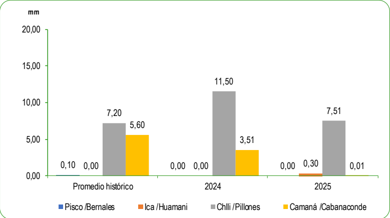
GRÁFICO N°70 PERÚ: PROMEDIO DE LAS PRECIPITACIONES EN LA ZONA SUR DE LA VERTIENTE DEL PACÍFICO OCTUBRE 2024 - 2025 Milímetros (mm)
