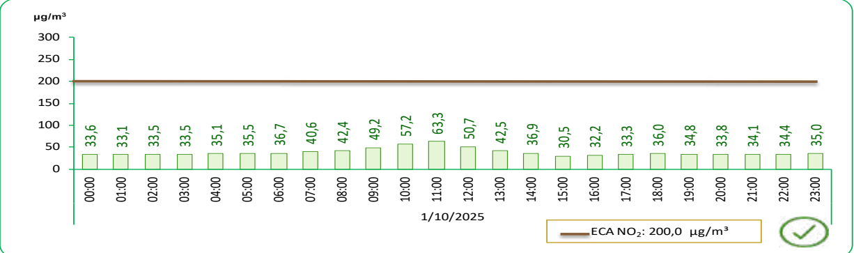
GRÁFICO N°25 LIMA METROPOLITANA: VALOR DIARIO DEL DIÓXIDO DE NITRÓGENO (NO 2 ), EN LA ESTACIÓN DE MEDICIÓN DE CERES – OCTUBRE 2025
