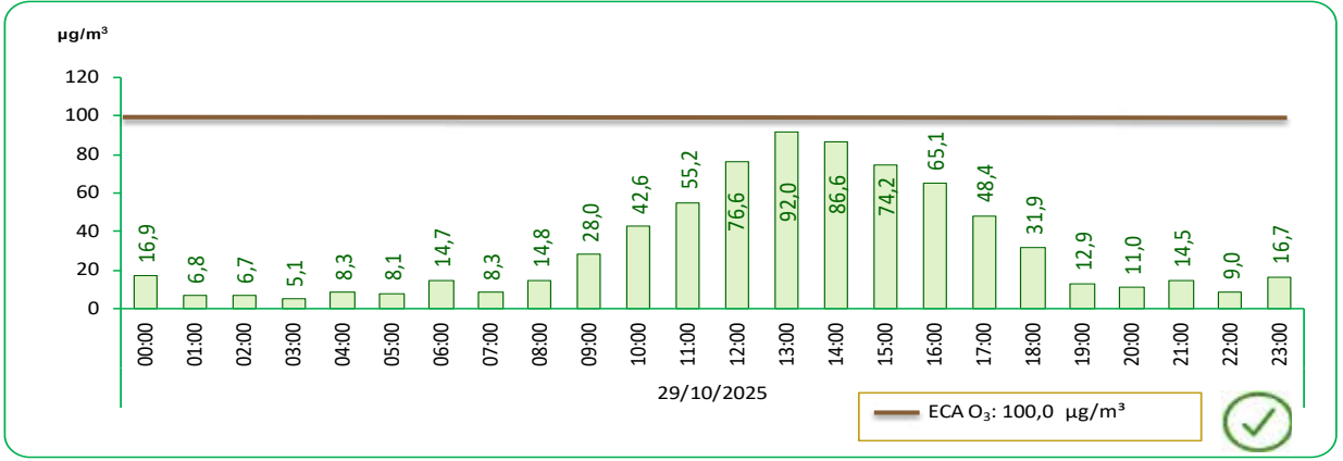
GRÁFICO N°43 LIMA METROPOLITANA: VALOR DIARIO DEL OZONO TROPOSFÉRICO (O 3 ), EN LA ESTACIÓN DE MEDICIÓN DE VILLA MARIA DEL TRIUNFO – OCTUBRE 2025
