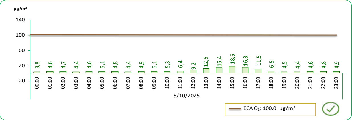
GRÁFICO N°42 LIMA METROPOLITANA: VALOR DIARIO DEL OZONO TROPOSFÉRICO (O 3 ), EN LA ESTACIÓN DE MEDICIÓN DE PARIACHI – OCTUBRE 2025
