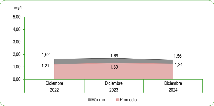
GRÁFICO N°54 LIMA METROPOLITANA: CONCENTRACIÓN DE MATERIA ORGÁNICA EXPRESADA COMO TOC EN LAS PLANTAS DE TRATAMIENTO 1 Y 2 DE SEDAPAL Mes: Diciembre 2022 - 2024 Miligramos por litro (mg/l)
