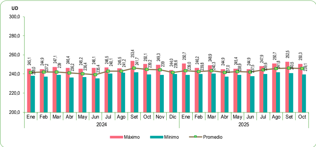
GRÁFICO N°44 PERÚ: VIGILANCIA DEL OZONO ATMOSFÉRICO EN LA ESTACIÓN VAG MARCAPOMACOA OCTUBRE 2025 – OCTUBRE2024 Unidades Dobson (UD)
