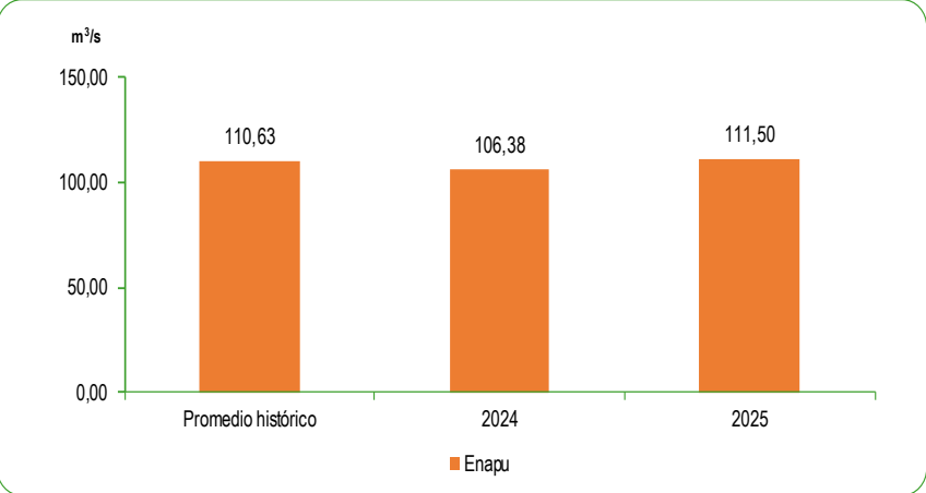
GRÁFICO N°64 PERÚ: CAUDAL PROMEDIO DE LOS RÍOS DE LA ZONA NORTE DE LA VERTIENTE DEL ATLÁNTICO OCTUBRE 2024 – 2025 Metro cúbico por segundo (m³/s)
