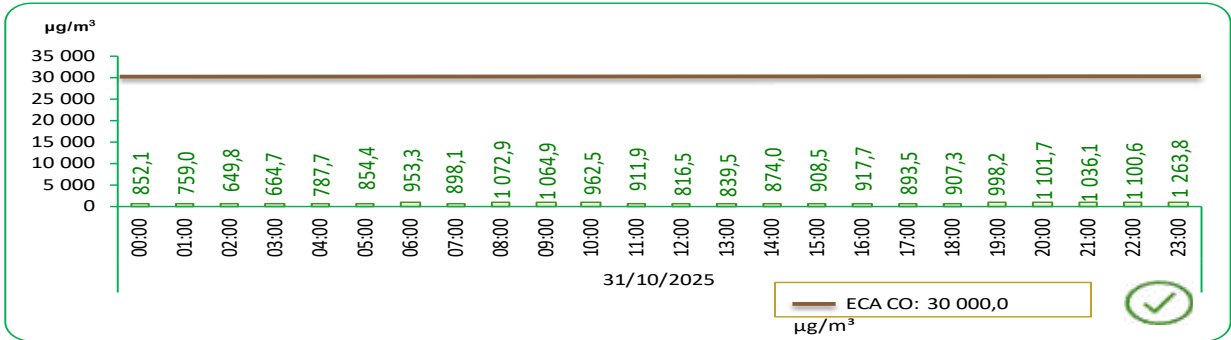
GRÁFICO N°31 LIMA METROPOLITANA: VALOR DIARIO DEL MONÓXIDO DE CARBONO (CO), EN LA ESTACIÓN DE MEDICIÓN DE CAMPO DE MARTE – OCTUBRE 2025
