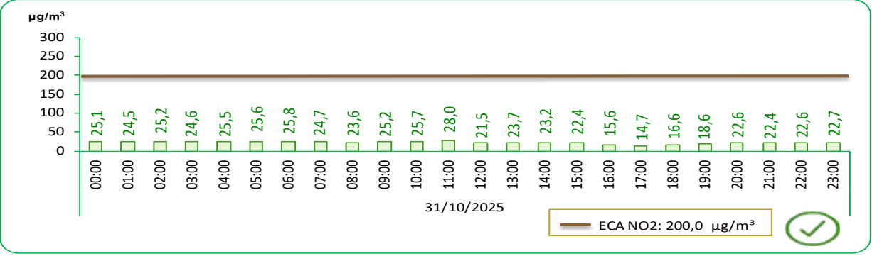
GRÁFICO N°26 LIMA METROPOLITANA: VALOR DIARIO DEL DIÓXIDO DE NITRÓGENO (NO 2 ), EN LA ESTACIÓN DE MEDICIÓN DE VILLA MARÍA DEL TRIUNFO – OCTUBRE 2025
