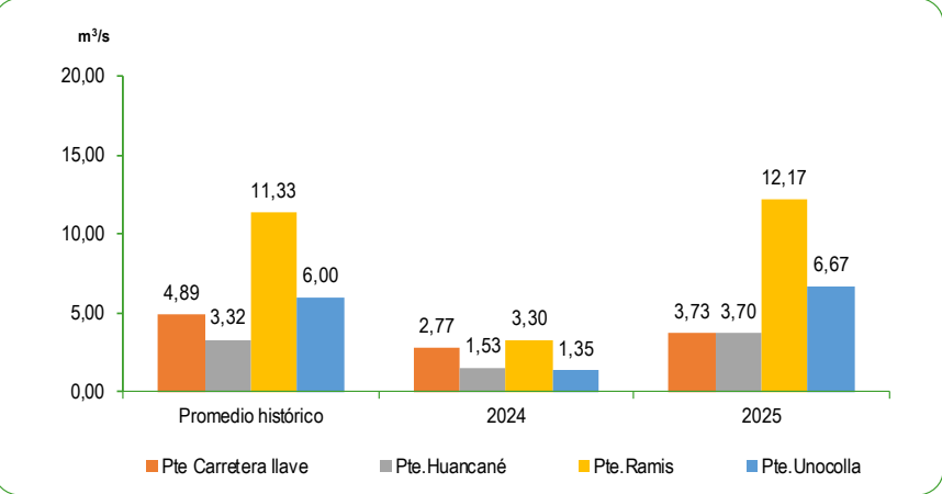
GRÁFICO N°67 PERÚ: CAUDAL PROMEDIO DE LOS RÍOS DE LA VERTIENTE DEL LAGO TITICACA OCTUBRE 2024 – 2025 Metro cúbico por segundo (m³/s)
