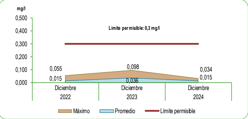
GRÁFICO N°46 LIMA METROPOLITANA: CONCENTRACIÓN DE HIERRO (Fe) EN LAS PLANTAS DE TRATAMIENTO 1 Y 2 DE SEDAPAL Mes: Diciembre 2022 - 2024 Miligramos por litro (mg/l)
