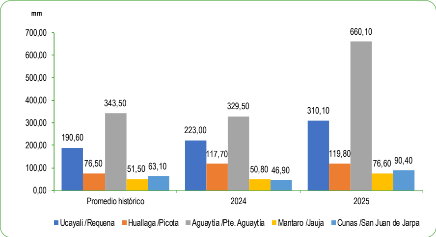
GRÁFICO N°72 PERÚ: PROMEDIO DE LAS PRECIPITACIONES EN LA ZONA CENTRO DE LA VERTIENTE DEL ATLÁNTICO OCTUBRE 2024 – 2025 Milímetros (mm)
