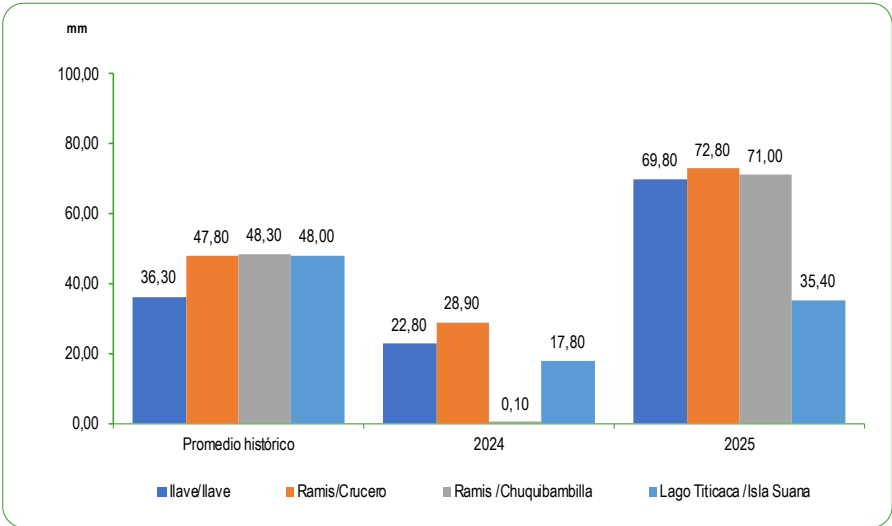
GRÁFICO N°74 PERÚ: PROMEDIO DE LAS PRECIPITACIONES EN LA VERTIENTE DEL LAGO TITICACA OCTUBRE 2024 – 2025 Milímetros (mm)
