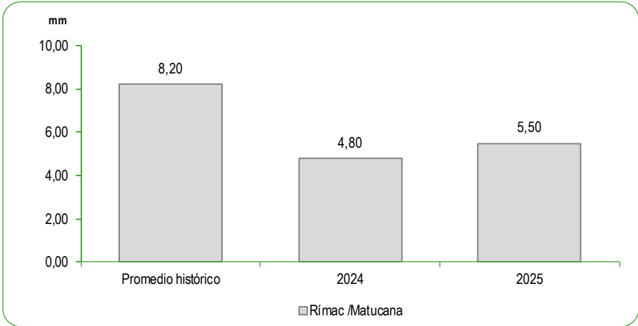
GRÁFICO N°69 PERÚ: PROMEDIO DE LAS PRECIPITACIONES EN LA ZONA CENTRO DE LA VERTIENTE DEL PACÍFICO OCTUBRE 2024 – 2025 Milímetros (mm)
