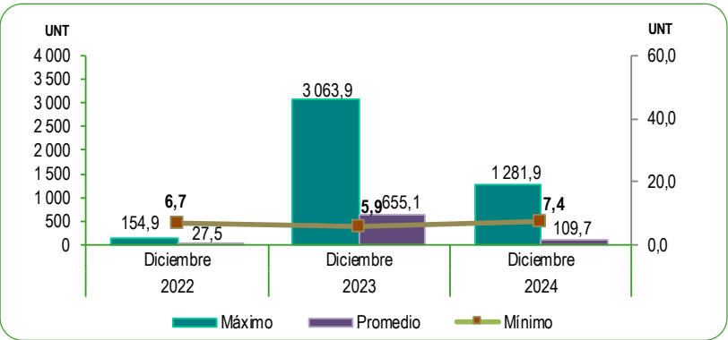
GRÁFICO N°57 LIMA METROPOLITANA: NIVELES DE TURBIEDAD EN EL RÍO RÍMAC Mes: Diciembre 2022 - 2024 Unidades Nefelométricas de Turbiedad (UNT)
