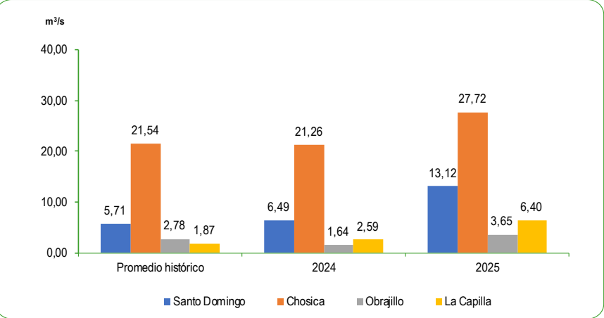
GRÁFICO N°62 PERÚ: CAUDAL PROMEDIO DE LOS RÍOS DE LA ZONA CENTRO DE LA VERTIENTE DEL PACÍFICO OCTUBRE 2024 – 2025 Metro cúbico por segundo (m³/s)
