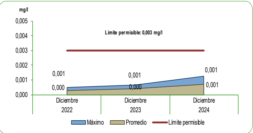
GRÁFICO N°50 LIMA METROPOLITANA: CONCENTRACIÓN DE CADMIO (Cd) EN LAS PLANTAS DE TRATAMIENTO 1 Y 2 DE SEDAPAL Mes: Diciembre 2022 - 2024 Miligramos por litro (mg/l)
