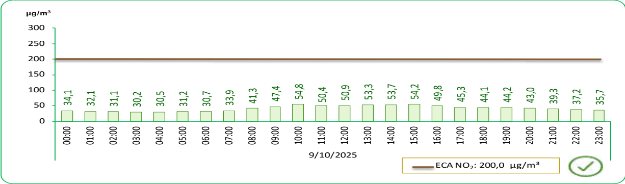
GRÁFICO N°24 LIMA METROPOLITANA: VALOR DIARIO DEL DIÓXIDO DE NITRÓGENO (NO 2 ), EN LA ESTACIÓN DE MEDICIÓN DE SAN JUAN DE LURIGANCHO – OCTUBRE 2025
