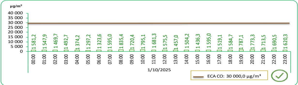
GRÁFICO N°30 LIMA METROPOLITANA: VALOR DIARIO DEL MONÓXIDO DE CARBONO (CO), EN LA ESTACIÓN DE MEDICIÓN DE SAN BORJA – OCTUBRE 2025
