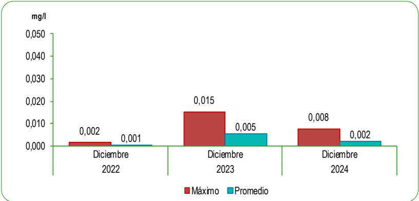
GRÁFICO N°45 LIMA METROPOLITANA: CONCENTRACIÓN DE CADMIO (Cd) EN EL RÍO RÍMAC Mes: Diciembre 2022 - 2024 Miligramos por litro (mg/l)
