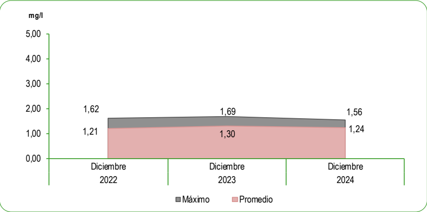
GRÁFICO N°50 LIMA METROPOLITANA: CONCENTRACIÓN DE MATERIA ORGÁNICA EXPRESADA COMO TOC EN LAS PLANTAS DE TRATAMIENTO 1 Y 2 DE SEDAPAL Mes: Diciembre 2022 - 2024 Miligramos por litro (mg/l)
