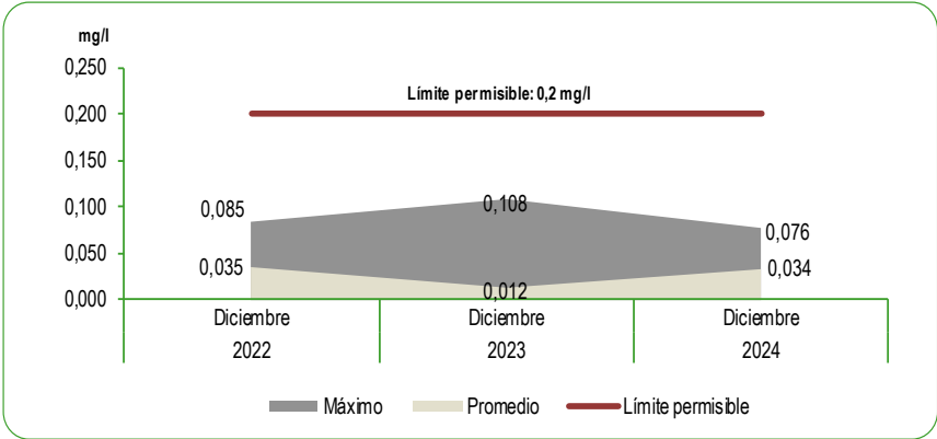
GRÁFICO N° 48 LIMA METROPOLITANA: CONCENTRACIÓN DE ALUMINIO (Al) EN LAS PLANTAS DE TRATAMIENTO 1 Y 2 DE SEDAPAL Mes: Diciembre 2022 - 2024 Miligramos por litro (mg/l)
