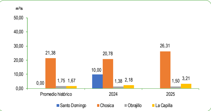
GRÁFICO N°58 PERÚ: CAUDAL PROMEDIO DE LOS RÍOS DE LA ZONA CENTRO DE LA VERTIENTE DEL PACÍFICO JULIO 2024 – 2025 Metro cúbico por segundo (m³/s)
