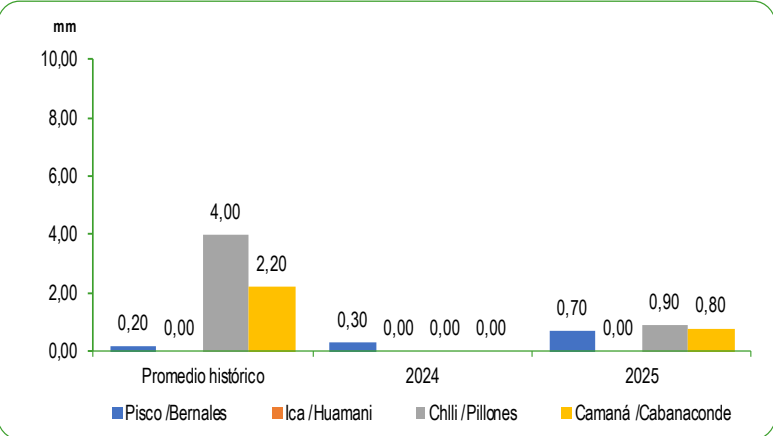
GRÁFICO N°66 PERÚ: PROMEDIO DE LAS PRECIPITACIONES EN LA ZONA SUR DE LA VERTIENTE DEL PACÍFICO JULIO 2024 - 2025 Milímetros (mm)
