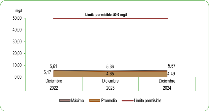
GRÁFICO N°52 LIMA METROPOLITANA: CONCENTRACIÓN DE NITRATOS (NO 3 ) EN LAS PLANTAS DE TRATAMIENTO 1 Y 2 DE SEDAPAL Mes: Diciembre 2022 - 2024 Miligramos por litro (mg/l)
