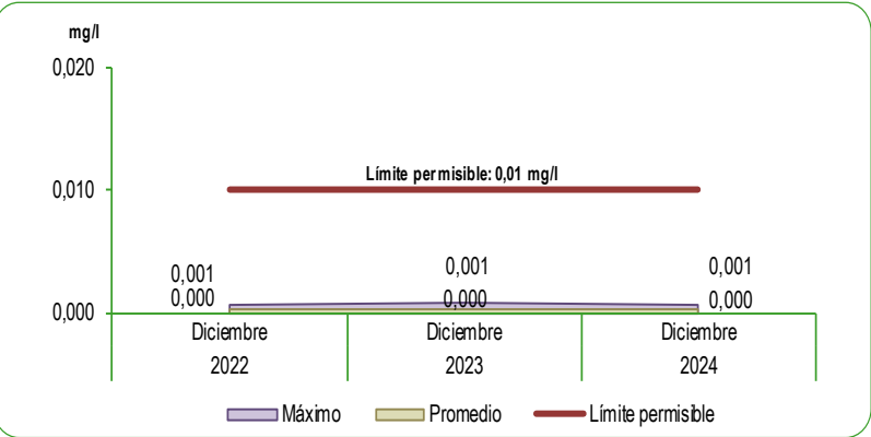
GRÁFICO N°44 LIMA METROPOLITANA: CONCENTRACIÓN DE PLOMO (Pb) EN LAS PLANTAS DE TRATAMIENTO 1 Y 2 DE SEDAPAL Mes: Diciembre 2022 - 2024 Miligramos por litro (mg/l)
