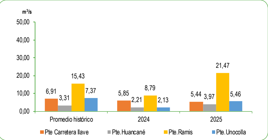
GRÁFICO N°63 PERÚ: CAUDAL PROMEDIO DE LOS RÍOS DE LA VERTIENTE DEL LAGO TITICACA JULIO 2024 – 2025 Metro cúbico por segundo (m³/s)
