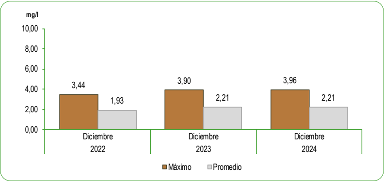
GRÁFICO N°49 LIMA METROPOLITANA: CONCENTRACIÓN DE MATERIA ORGÁNICA EXPRESADA COMO TOC EN EL RÍO RÍMAC Mes: Diciembre 2022 - 2024 Miligramos por litro (mg/l)
