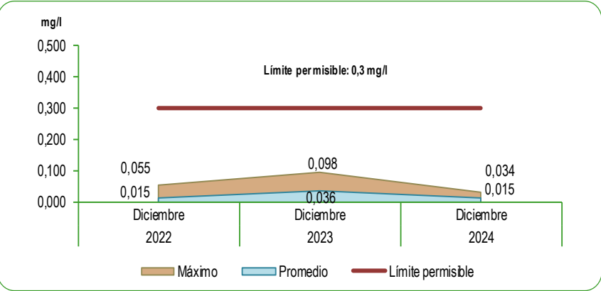
GRÁFICO N°42 LIMA METROPOLITANA: CONCENTRACIÓN DE HIERRO (Fe) EN LAS PLANTAS DE TRATAMIENTO 1 Y 2 DE SEDAPAL Mes: Diciembre 2022 - 2024 Miligramos por litro (mg/l)
