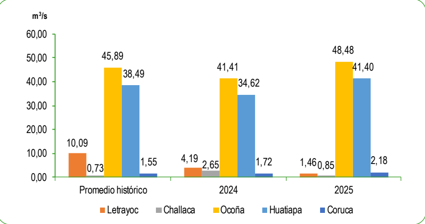
GRÁFICO N°59 PERÚ: CAUDAL PROMEDIO DE LOS RÍOS DE LA ZONA SUR DE LA VERTIENTE DEL PACÍFICO JULIO 2024 – 2025 Metro cúbico por segundo (m³/s)
