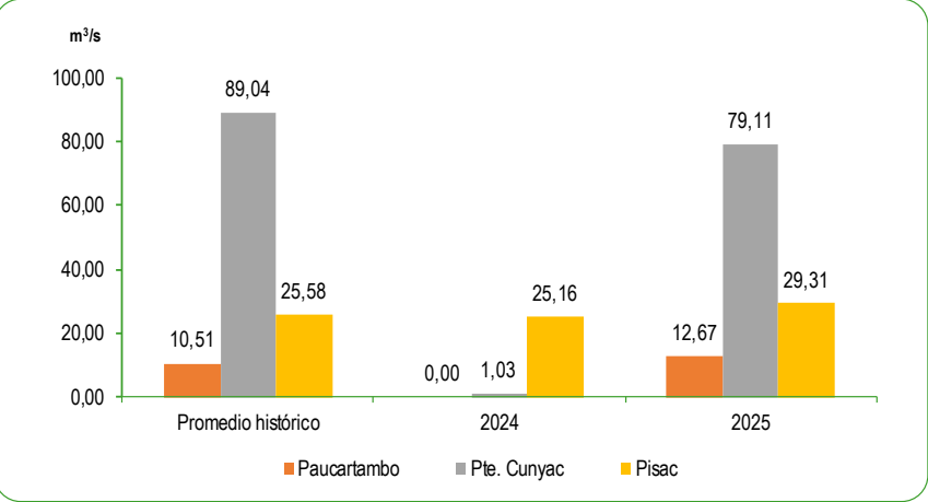
GRÁFICO N°62 PERÚ: CAUDAL PROMEDIO DE LOS RÍOS DE LA ZONA SUR DE LA VERTIENTE DEL ATLÁNTICO JULIO 2024 – 2025 Metro cúbico por segundo (m³/s)
