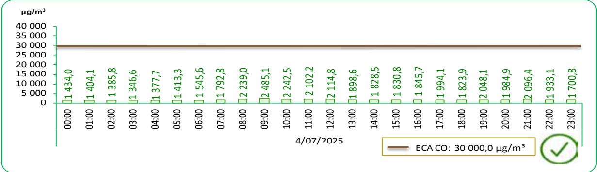
GRÁFICO N°30 LIMA METROPOLITANA: VALOR DIARIO DEL MONÓXIDO DE CARBONO (CO), EN LA ESTACIÓN DE MEDICIÓN DE SAN BORJA – JULIO 2025
