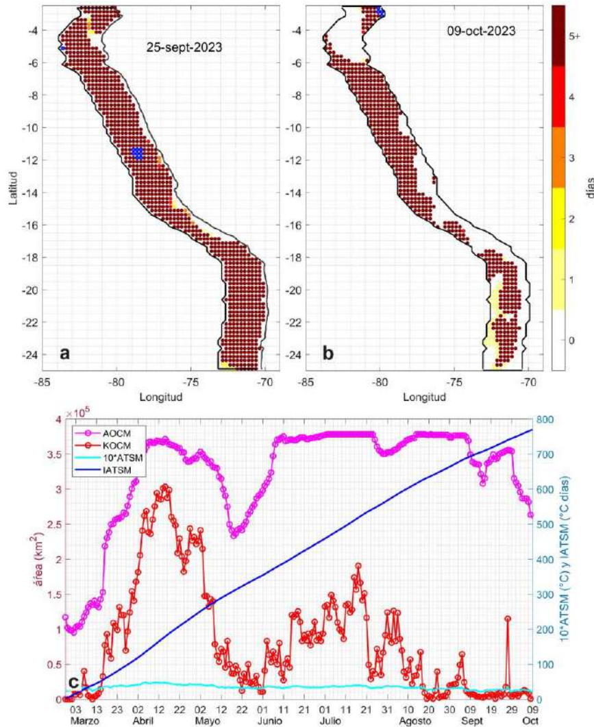
Figura 16. Extensión de la ola de calor marina (OCM) dentro de la franja de 150 millas frente a la costa el 25 de septiembre (a) y el 8 de octubre del 2023 (b); la escala de color indica el número de días en los cuales la TSM superó el percentil 90 de los datos diarios históricos, usando el período 1982-2011 como referencia (Pietri et al., 2021); los círculos con relleno azul indican que allí la OCM supera la anomalía de +4 °C; c) Series de tiempo de indicadores de la OCM para la zona entre los 2 y 15° S y dentro de las 150 mn: área de la OCM (AOCM, Km 2 ); área de la OCM donde la ATSM > +4 °C (KOCM, Km 2 ); anomalía diaria de la TSM; y anomalía integrada (IATSM; °C x días). En promedio, la ATSM en la OCM desde el 1 de abril hasta el 8 de mayo fue +4,3 °C. Fuente: OISST 2.1; procesamiento: IMARPE.
