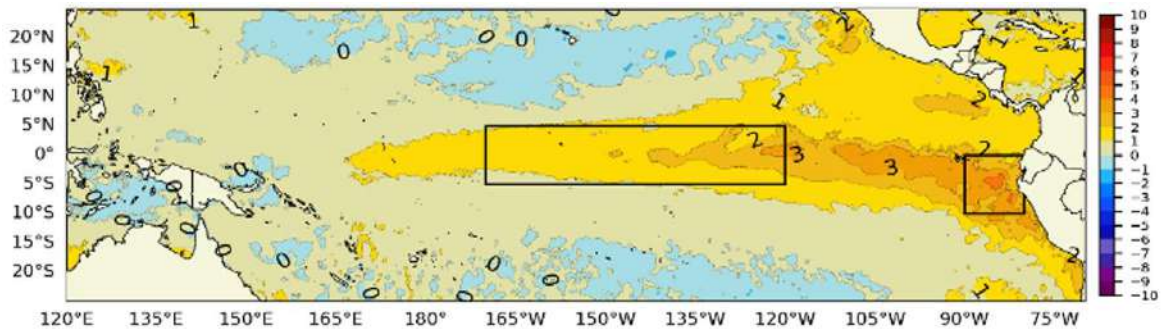
Figura 1. Promedio de las anomalías de la TSM en el Pacífico tropical del 16 al 30 de setiembre. Fuente: OSTIA. Procesamiento: DIHIDRONAV.
