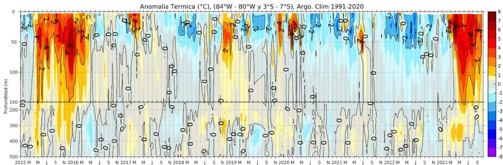
Figura 24. Anomalia térmica en base a los perfiladores ARGO, frente al zona norte; climatología: 1991 - 2020 (Domínguez et al., 2023)
