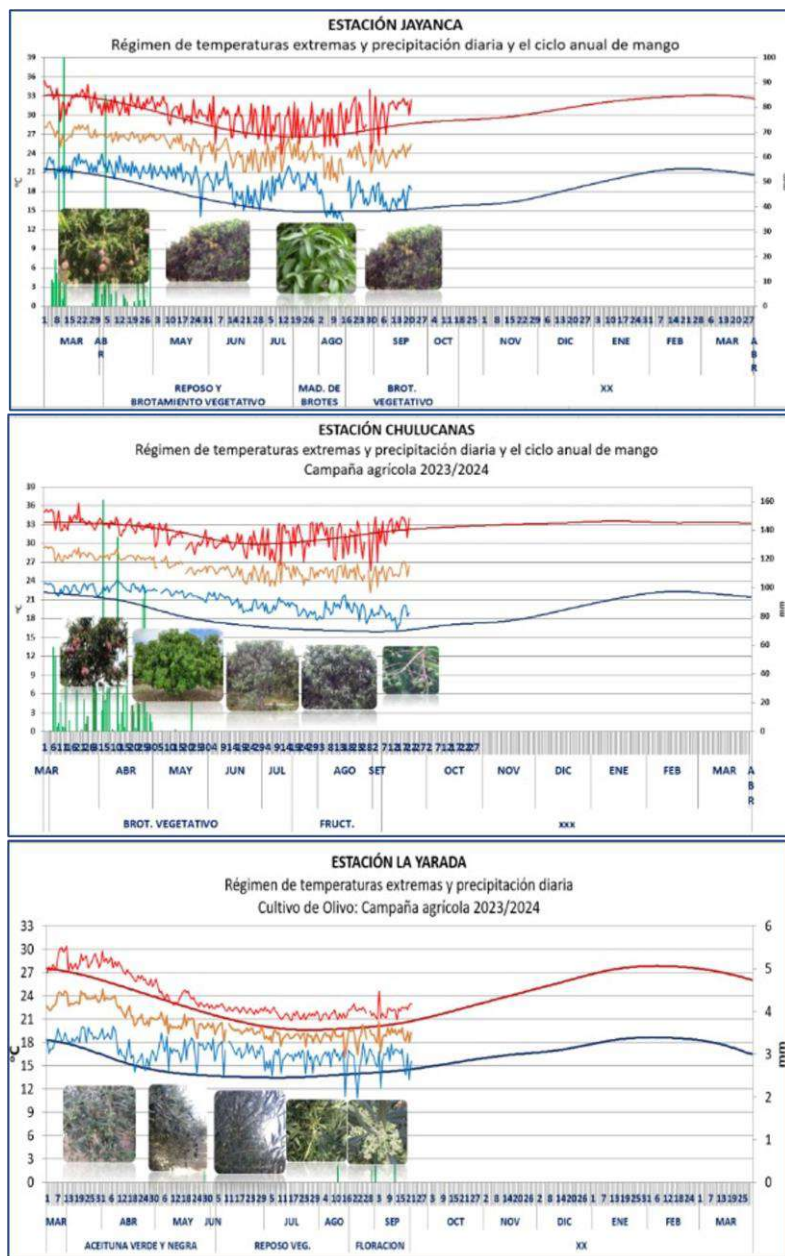
Figura 38. Monitoreo agrometeorológico del mango y el olivo campañas agrícolas 2023/2024 en las estaciones de Jayanca, Chulucanas y La Yarada. Fuente: SENAMHI.
