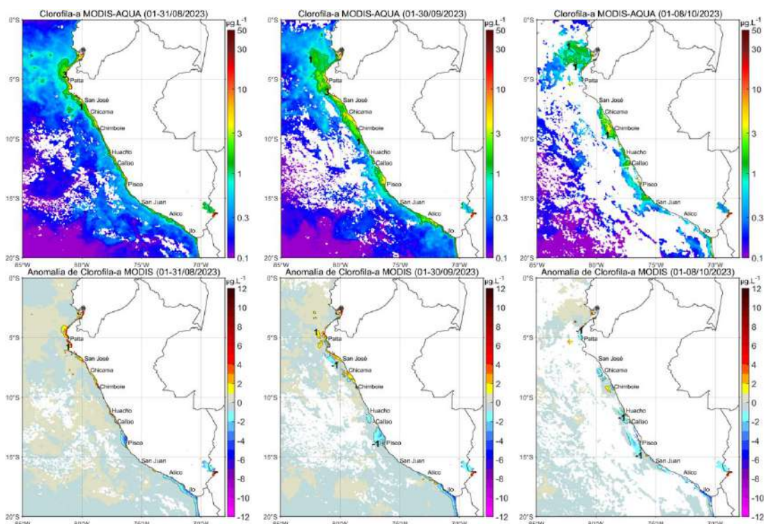
Figura 27. Distribución de la concentración de clorofila-a superficial satelital ( \mu\text{g L}^{-1} , panel superior) y su anomalía ( \mu\text{g L}^{-1} , panel inferior), durante mayo, setiembre y lo que va de octubre de 2023 (de izquierda a derecha), proveniente de MODIS-AQUA. Fuente: Fuente: Satélite MODIS. Procesamiento: LHQ/AFIOQG/DGIOCC/IMARPE.
