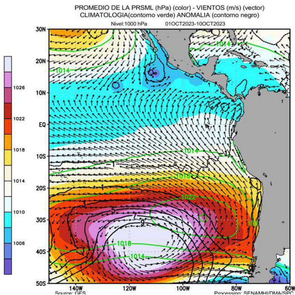
Figura 7. Promedio entre el 1 y el 10 de octubre del 2023 de la presión atmosférica a nivel del mar (sombreado), anomalía de la presión atmosférica (líneas negras) y valor climatológico (líneas verdes). Viento en 1000 hPa superiores a los 2 m/s (vectores). Fuente: GFS. Procesamiento: SENAMHI
