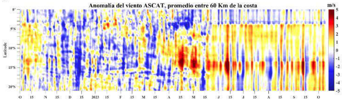
Figura 11. Viento satelital (40 Km frente a la costa del Perú): a) Velocidad del viento ( \text{m s}^{-1} ), b) Anomalia de la velocidad del viento ( \text{m s}^{-1} ). Fuente: Satélite ASCAT + GFS (desde 21 de mayo), Procesamiento: Laboratorio de Hidro-Física Marina y Laboratorio Costero de Santa Rosa, IMARPE. Climatología 2000 – 2014. Actualizado al 10 de octubre.
