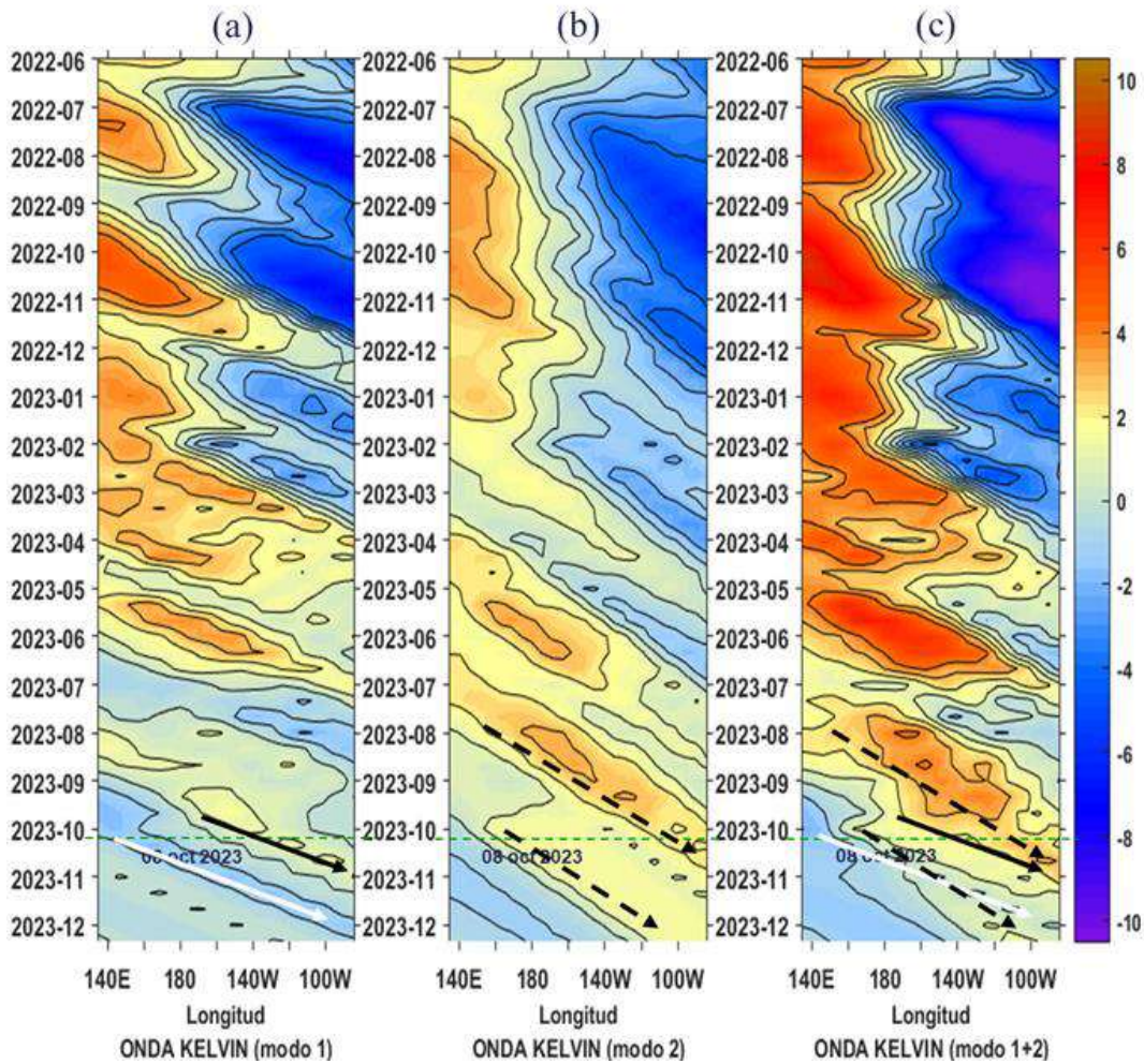
Figura 41. Diagrama Hovmöller longitud-tiempo de las ondas Kelvin en el océano Pacífico ecuatorial (0°N): (a) Modo 1 (flechas con líneas continuas), (b) Modo 2 (flechas con líneas discontinuas), (c) Modos 1+2. Se presentan las ondas de hundimiento “cálidas” (flechas negras), y las ondas de afloramiento “frías” (flechas blancas). La línea discontinua horizontal, en verde, indica el inicio del pronóstico con el forzante de vientos climatológico. Fuente: IMARPE, forzado con anomalías del esfuerzo de vientos de NCEP. Procesamiento: LMOECC/AFIOF/DGIOCC/IMARPE.
