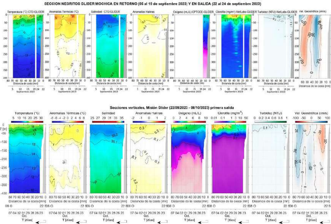
Figura 21. Secciones verticales de temperatura (°C), anomalías térmicas (°C), salinidad, anomalías halinas, oxígeno (mL L -1 ), clorofila (mg m -3 ), turbidez (NTU) y corrientes geostóricas (cm s -1 ), a partir de los datos registrados por el glider Mochica frente a Negritos – Talara (entrada y salida), registrados desde el 05 de setiembre hasta el 08 de octubre.
