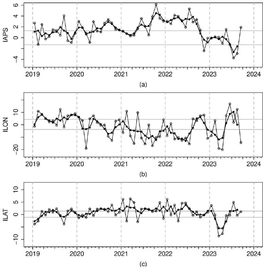
Figura 10. Variación temporal de los índices del APS: a) índice de intensidad (IAPS) e índices de posición b) longitudinal (ILON) y c) latitudinal (ILAT) hasta el trimestre JAS 2023 (círculos negros). Los círculos blancos indican las anomalías mensuales en el periodo enero 2019 hasta setiembre 2023.
