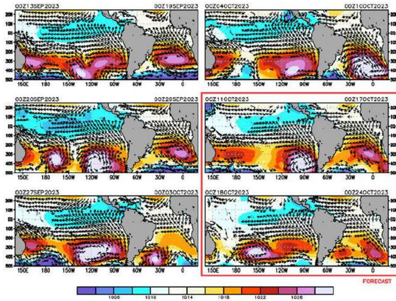
Figura 8. Promedio semanal de la presión atmosférica reducida a nivel del mar (colores) y vientos (flechas). Análisis: del 13 de setiembre al 10 de octubre de 2023. Pronóstico: del 11 de octubre al 24 de octubre de 2023 Fuente: GFS. Procesamiento: SENAMHI
