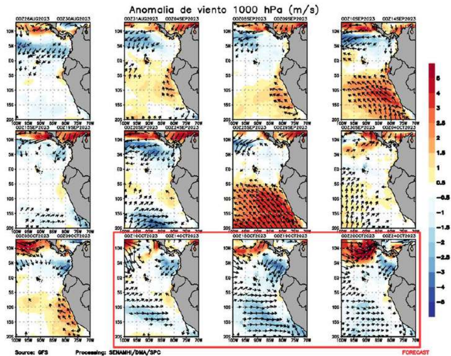
Figura 9. Anomalia pentadal del viento (m/s) a 10 m de altura frente a la costa noroccidental de Sudamérica y Centroamérica. Fuente: GFS. Análisis: del 26 de agosto al 09 de octubre de 2023. Pronóstico: del 10 al 24 de octubre de 2023. Procesamiento: SENAMHI.
