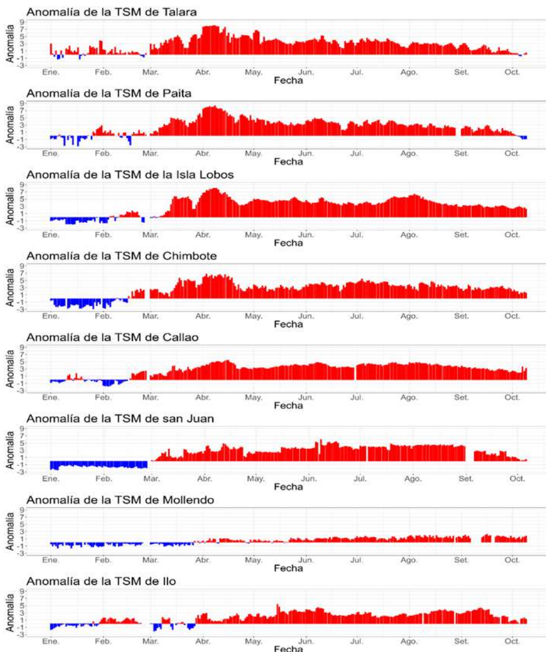
Figura 15. Anomalía de la TSM diaria a lo largo del litoral de Perú de enero a octubre 2023. Climatología: 1991-2020. Fuente y procesamiento: DIHIDRONAV.
