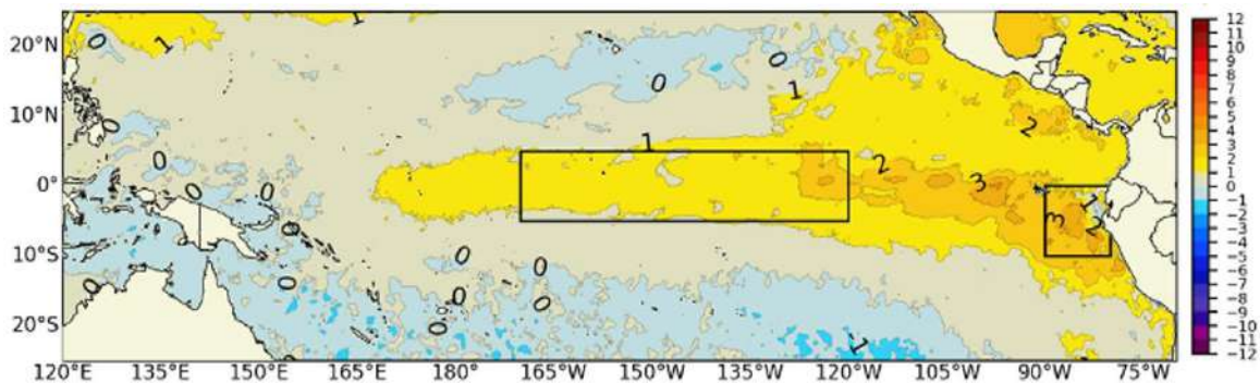
Figura 2. Promedio de las anomalías de la TSM en el Pacífico del 01 al 09 de octubre de 2023. Fuente: OSTIA. Procesamiento: DIHIDRONAV
