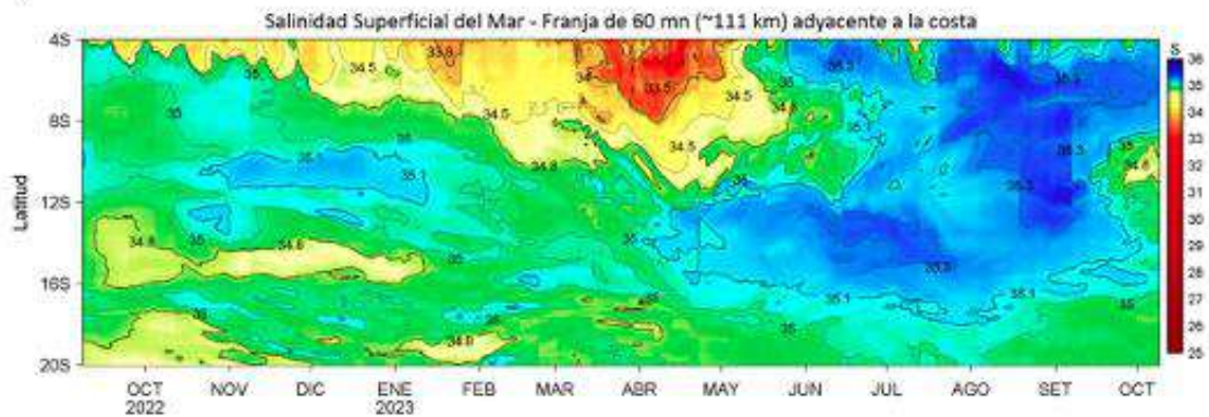
Figura 25. (a) Distribución quincenal de la Salinidad Superficial del Mar (SSM) en el Pacífico Sudeste, durante el mes de 7 de setiembre y 9 de octubre del 2023. (b) Diagrama Hovmöller de la SSM en la franja de las 60 millas costeras, al 9 de octubre de 2023. Datos: GLOBAL_ANALYSIS_FORECAST_PHY_001_024 (Lellouche, J.-M. et al, 2013) disponible en http://marine.copernicus.eu/services-portfolio/access-to-products/?option=com_csw&view=details&product_id=GLOBAL_ANALYSIS_FORECAST_PHY_001_024 . Procesamiento: LHF/AFIOF/DGIOCC/IMARPE.
