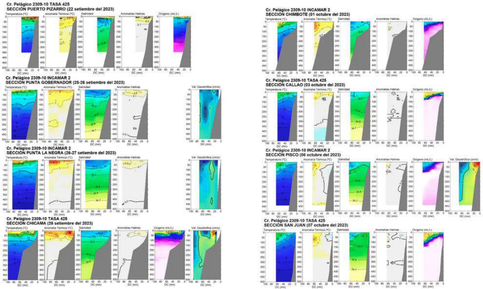
Figura 23. Secciones oceanográficas de temperatura, anomalía térmica, salinidad, anomalía halina, y oxígeno disuelto, realizadas frente a Puerto Pizarro, Punta Gobernador, Punta la Negra, Chicama, Chimbote y Callao dentro de las 100 mn, entre el 22 de septiembre y 03 de octubre de 2023. Climatología: 1991-2020 (Domínguez et al., 2023).
