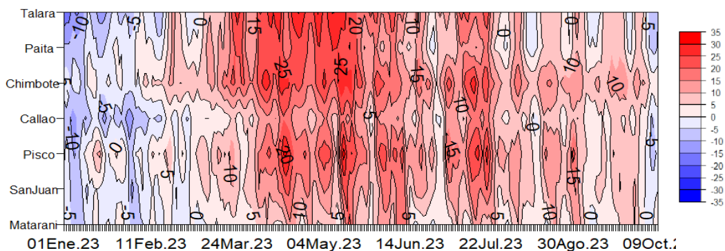
Figura 18. Diagrama Hovmöller de anomalía de NM en el litoral de Perú (con filtro móvil anual) del 1 de enero al 09 de octubre 2023, Climatología: 1991-2020. Procesamiento: DIHIDRONAV.
