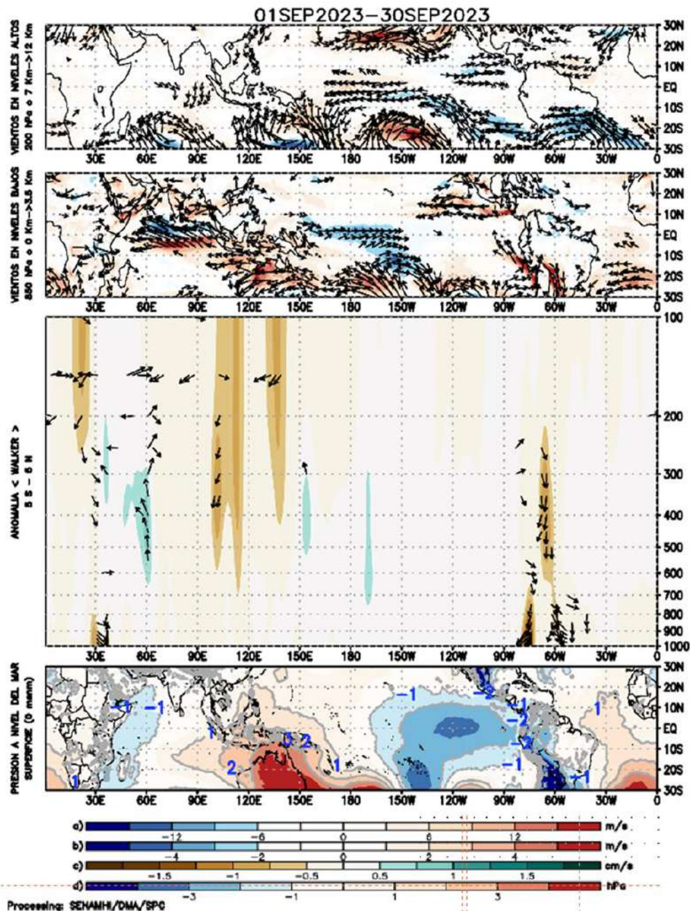
Figura 5. Análisis de la circulación atmosférica (Walker) entre el 1-30 de setiembre de 2023, (a) Anomalías de los vientos (colores) y su dirección (flechas) en niveles altos (200 hPa) y (b) bajos (850 hPa) de la atmósfera; c) Patrón anómalo de la circulación atmosférica ecuatorial (Walker), (d) Anomalías de presión a nivel del mar. Fuente: GFS. Procesamiento: SENAMHI
