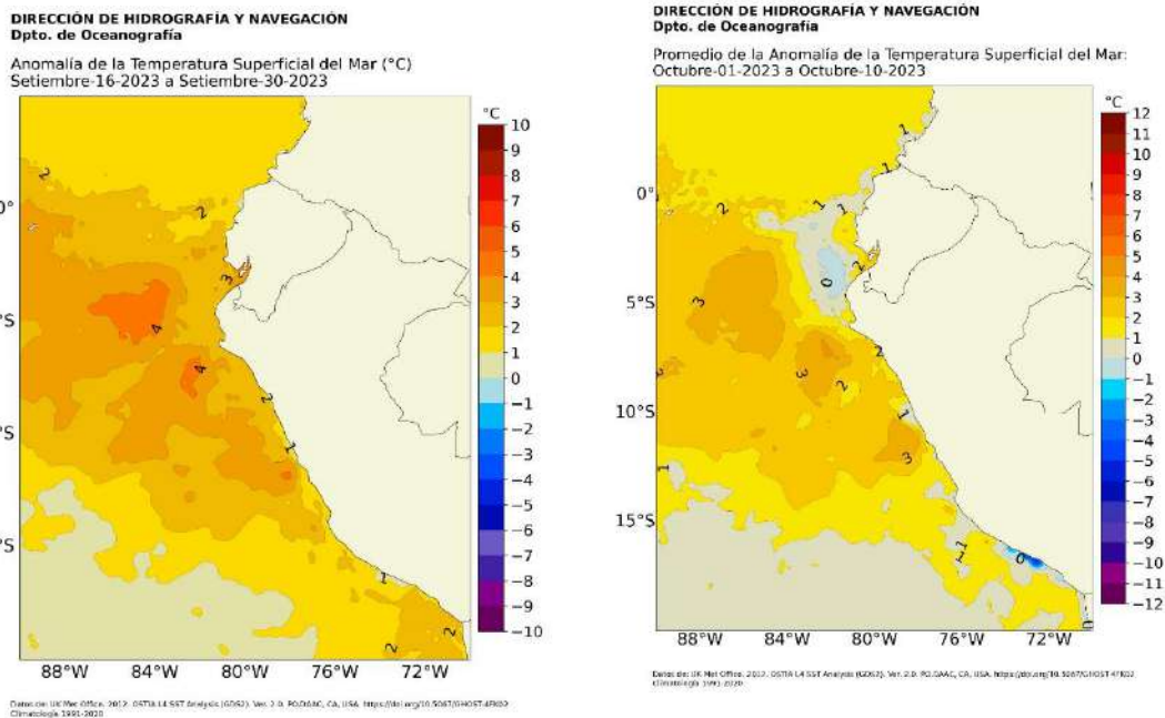
Figura 14. Carta de anomalías de la TSM en setiembre y octubre 2023, Climatología: 1991-2020. Fuente: OSTIA Procesamiento: DIHIDRONAV
