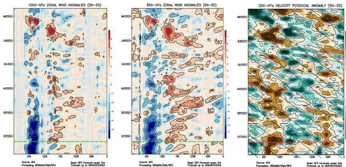
Figura 6. Anomalías promedio, ente los 5°N y 5°S de los (a) viento zonal en 1000 hPa y (b) viento zonal en 850 hPa y (c) velocidad potencial en 200 hPa. La línea verde muestra el inicio del periodo de pronóstico. Fuente: GFS. Procesamiento: SENAMHI
