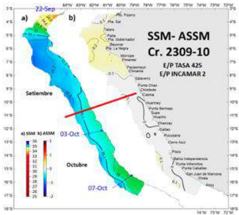
Figura 19. a) TSM (°C) y ATSM (°C) y b) SSM y ASSM, registrada durante el Crucero de Evaluación Hidroacústica de Recursos Pelágicos 23-10 del IMARPE. E/P TASA 425, E/P INCAMAR.
