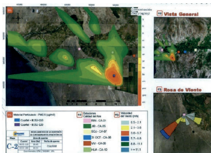
Figura 7. Simulación de concentración de contaminantes para el componente PM_{2.5} producto de la quema de caña de azúcar, correspondiente al 7 de noviembre del 2018
