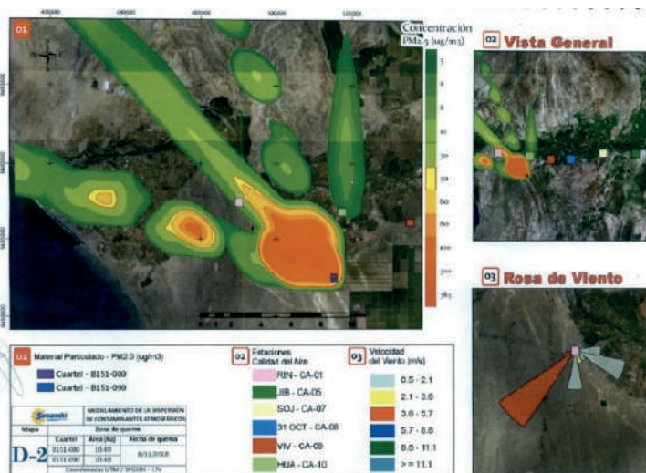
Figura 9. Simulación de concentración de contaminantes para el componente PM_{10} producto de la quema de caña de azúcar, correspondiente al 8 de noviembre del 2018
